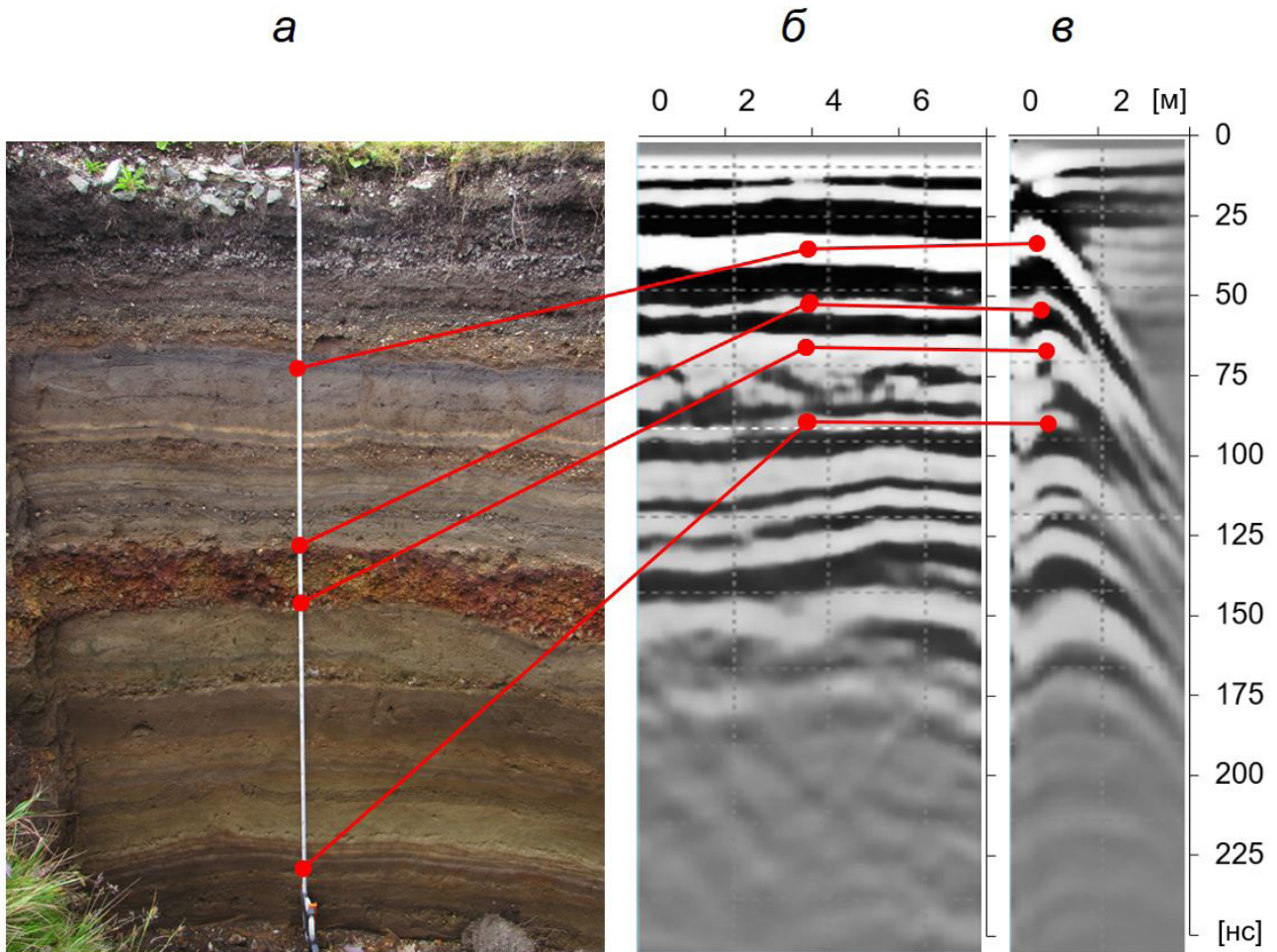
Рис. 4. Геологический разрез, полигон {01}: (а) — шурф, фотография; (б) — элемент георадарного профиля в районе шурфа; (в) — голограф, антенны 100 МГц. Прямыми выносными линиями указано соответствие физических границ раздела слоев геологического разреза осям синфазности георадиолокационного профиля и линиям голографа.
